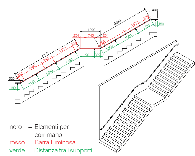
Disegno tecnico corrimano LaneLED INOX42
