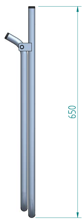
Ständer zugeklappt
