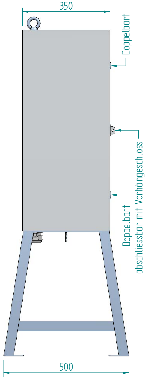
Schema Art.Nr. 231132
