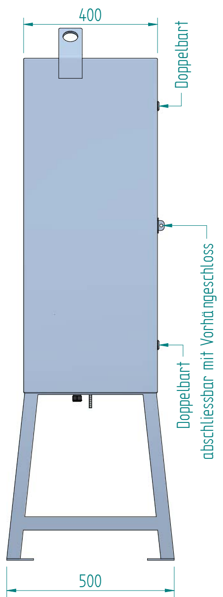
Schema Art.Nr. 231414
